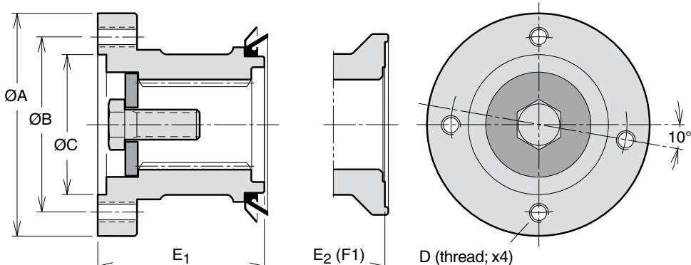
Fig. 4. SAE97 (370 4631) (378 0645)
