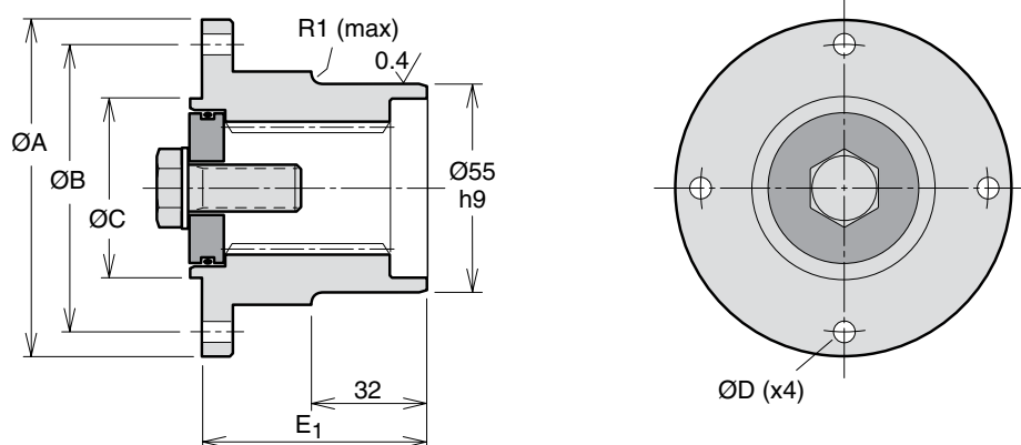
Fig. 2. DIN 90 (370 7423)
