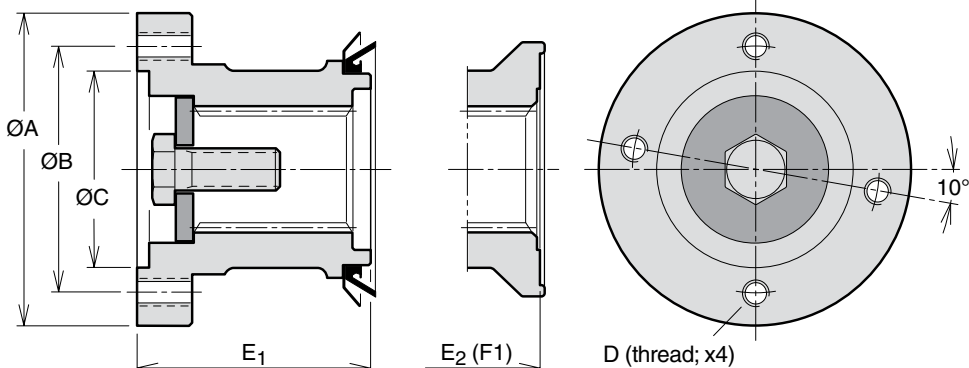
Fig. 3. SAE 88 (370 4628) (378 0644)
